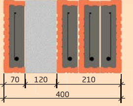
ZDIVO 400 mm
