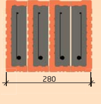
ZDIVO 300 mm
