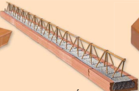
KMB KERAMICKÝ STROPNÍ NOSNÍK MIAKO
