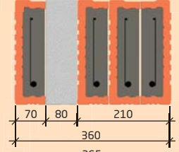
ZDIVO 365 mm
