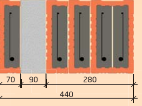
ZDIVO 440 mm
