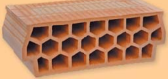
KMB MIAKO 19/62,5 250x525x190
